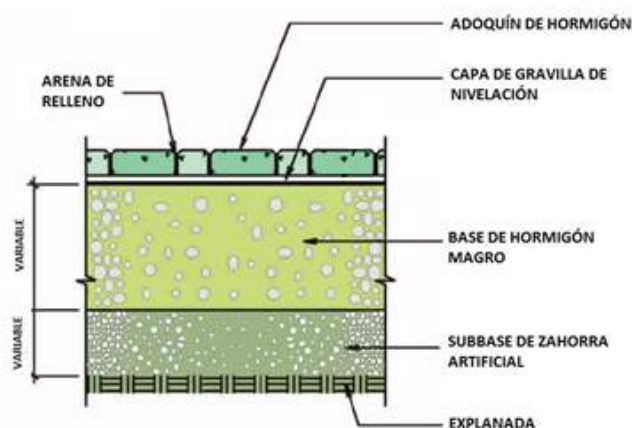
ILUSTRACIÓN 3. SECCIÓN TIPO DE PAVIMENTO CON ADOQUINES PARA VÍA PEATONAL
