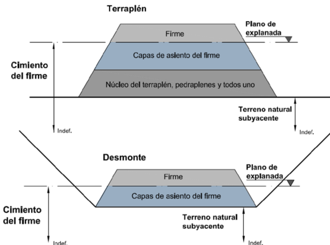
ILUSTRACIÓN 1. ESQUEMA DEL CIMIENTO DEL FIRME
